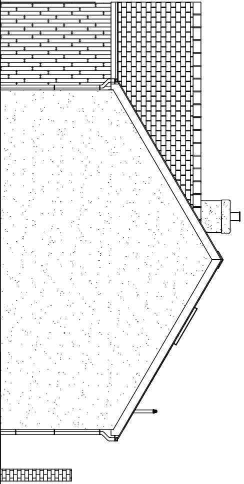
ELEVATION B
